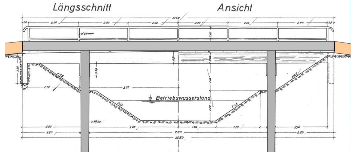
Prinzipskizze Überbauung
