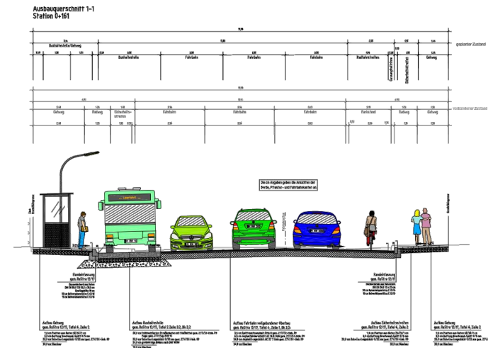
Regelprofil Straßenbau
