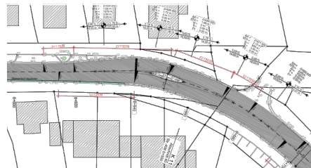
Lageplanausschnitt Straßenbau
