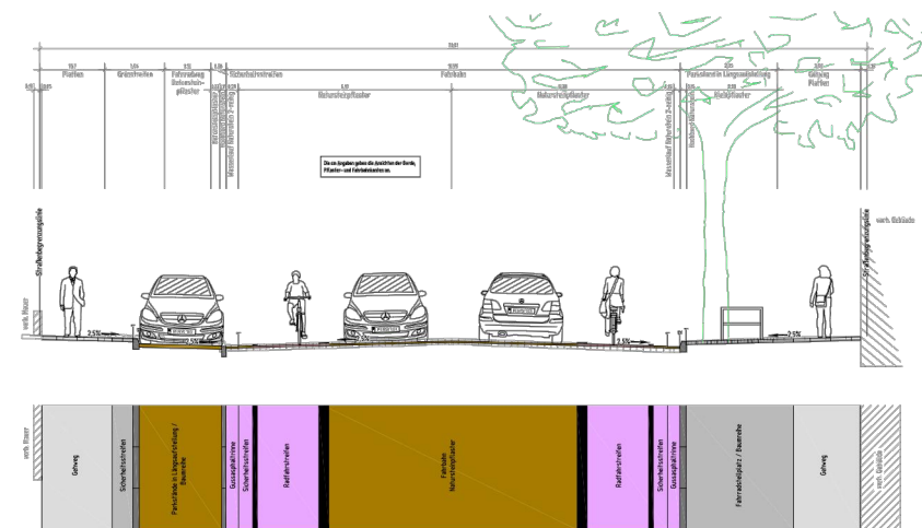
Regelprofil Straßenbau
